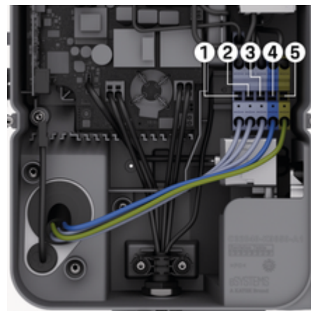
Kuva . 103: Liitäntäliittimet (3-vaiheinen)
