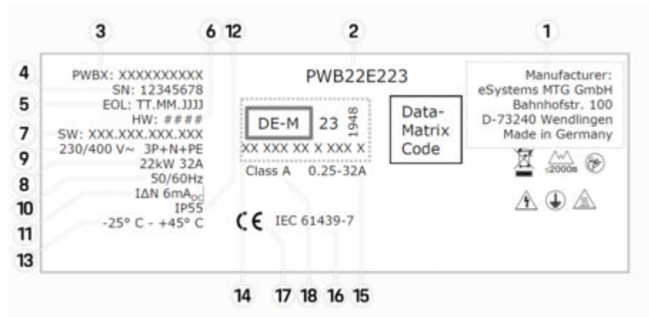
Fig. 90: Typeskilt (eksempel)
