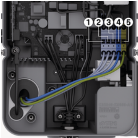
Fig. 53: Terminais (trifásicos)
