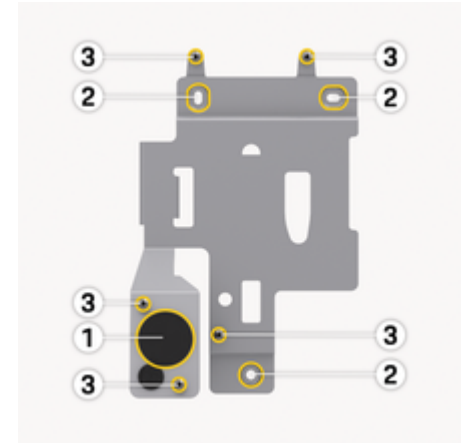
Abb. 2: Montageplatte
