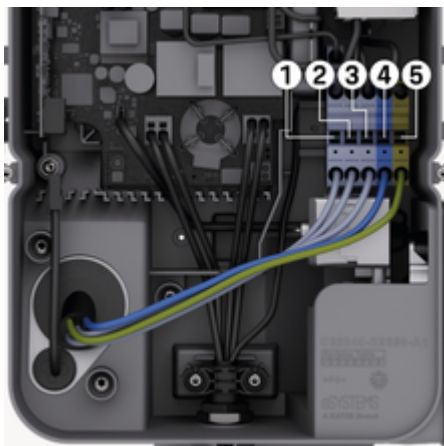
Rys. 143: Zaczepy przyłączeniowe (3-fazowe)
