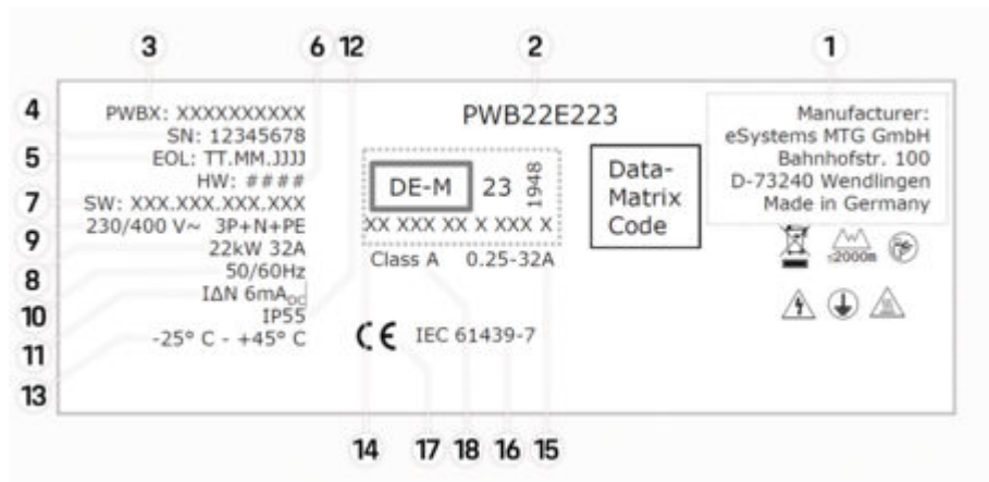
Εικ. 120: Πινάκίδα στοιχείων (παράδειγμα)
