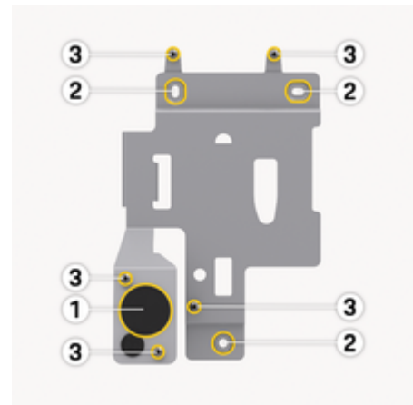
Afb. 72: Montageplaat
