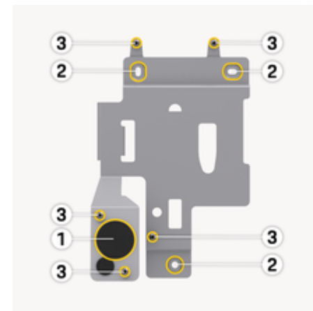
Rys. 142: Płyta montażowa
