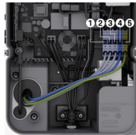
Obr. 123: Svorky (3fázové)
