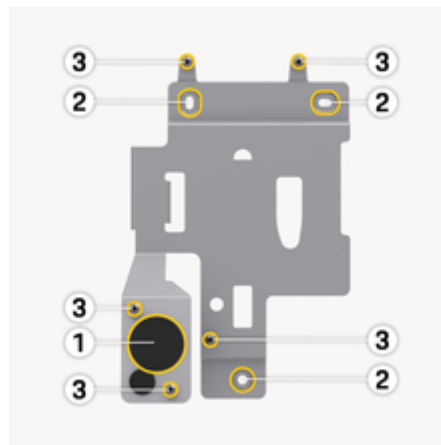
Bild 92: Monteringsplatta
