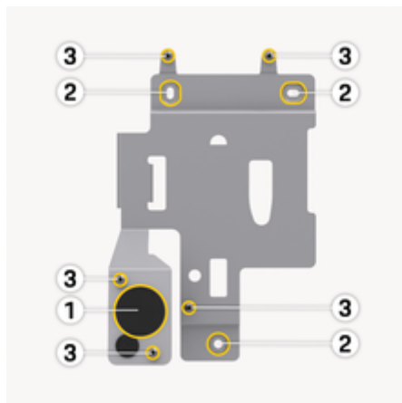
Obr. 122: Montážní deska
