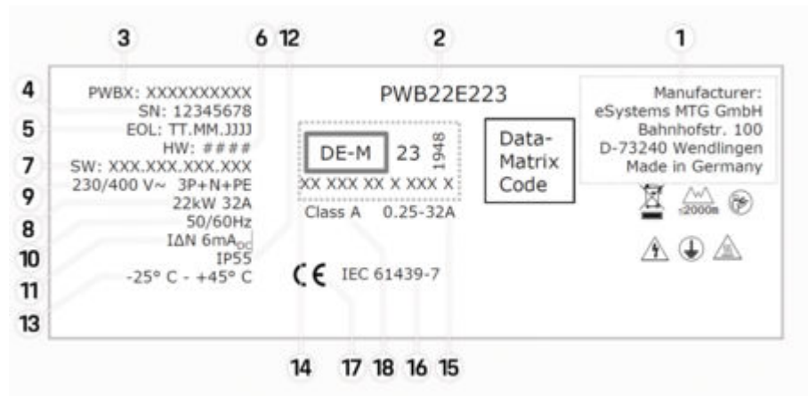
Abb. 10: Typenschild (Beispiel)
