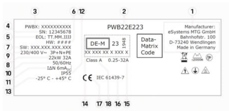
SI. 160: Tipaska tablica (primer)
