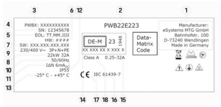
Bild 100: Typskylt (exempel)
