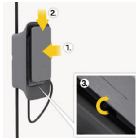
Sl. 158: Pritrjevanje sprednjega dela zasnove
