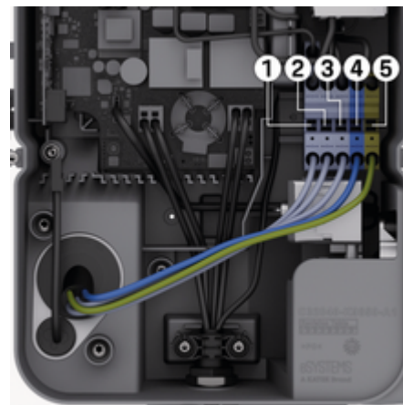
Bild 93: Kabelfästen (3-fas)
