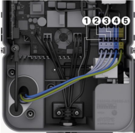
Afb. 73: Aansluitklemmen (3-fase)
