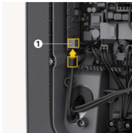
Bild 97: Fäst designramen
