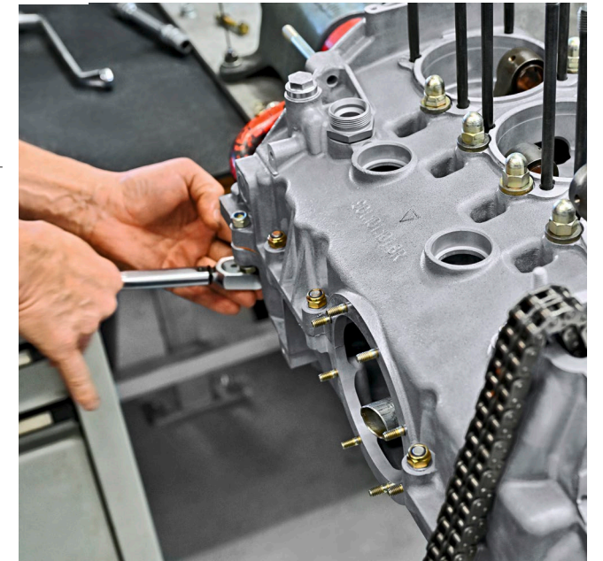
Bloc-moteur en magnésium 2,7 l Réf. 91110100145 Modèle 911 F (1973), uniquement pour 911 Carrera RS 2.7 Modèle 911 G (1974–1977), uniquement pour modèles à moteur de 2,7 l
