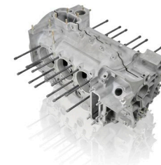
Bloc-moteur en magnésium 2,7 l Réf. 91110100145 Modèle 911 F (1973), uniquement pour 911 Carrera RS 2.7 Modèle 911 G (1974–1977), uniquement pour modèles à moteur de 2,7 l
