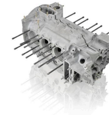
Bloc-moteur en magnésium 2,4 l Réf. 90110100147 Modèle 911 F (1972–1973), uniquement pour les véhicules à moteur de 2,4 l
