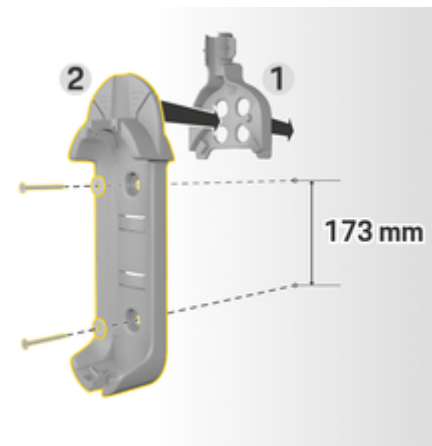
Fig. 6: Medidas de taladrado
