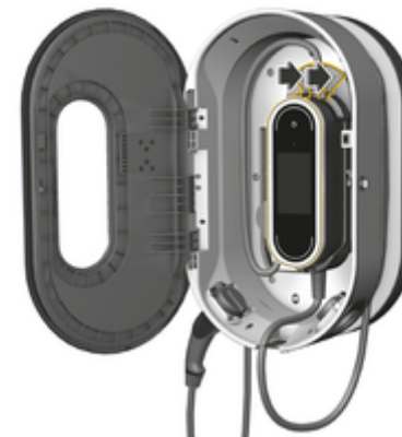
Fig. 20: Enganche la unidad de control
