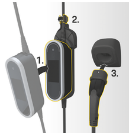
Fig. 9: Enganche la unidad de control
