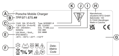
Abb. 11: Typenschild (Beispiel)
