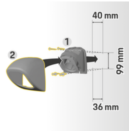
Abb. 5: Bohrmaße
