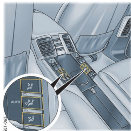
风量分配，后部控制面板（四区域空调系统）
