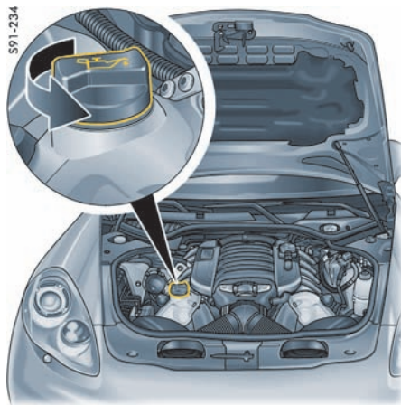
机油加注点（非 Panamera S Hybrid）
