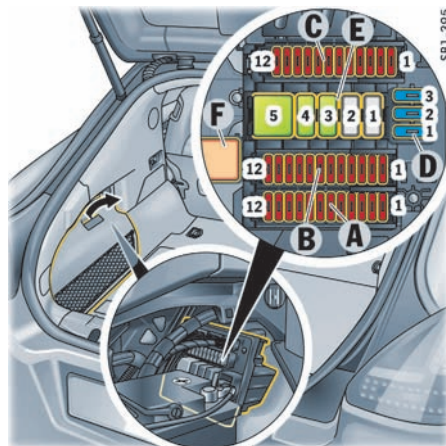
Panamera S Hybrid 行李厢内的保险丝 / 继电器盒：
