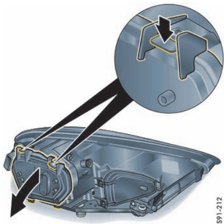
更换静态弯道灯 / 辅助远光灯灯泡
