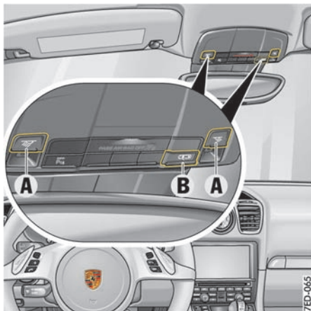
A - 车内灯 / 阅读灯按钮 B - 开启和关闭车内灯 / 阅读灯
