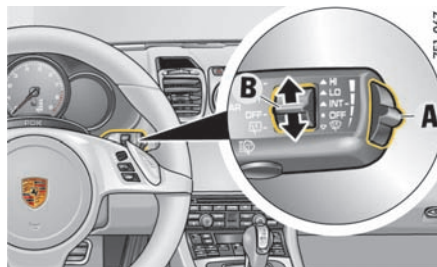
雨量传感器灵敏度 / 间歇式操作 (A) 和后雨刷器 (B) 的切换开关
