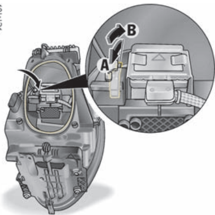
右侧大灯
