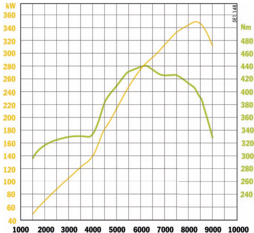
发动机全负荷曲线图
