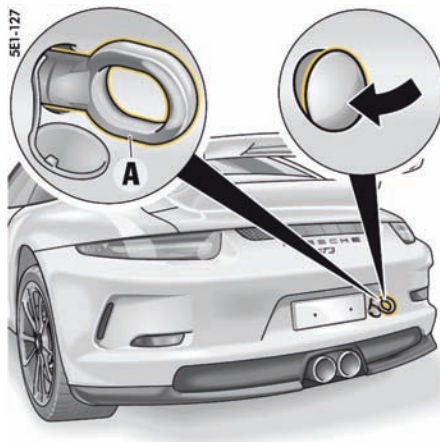
后牵引凸耳
