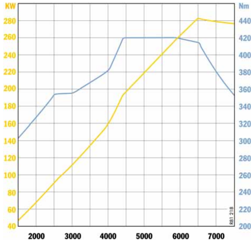
MA 101, 节气门全开时的发动机图谱, 911 Carrera S、911 Carrera 4S、911 Targa 4S
