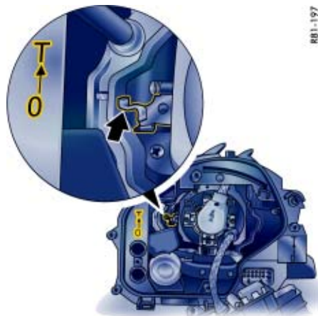
带弯道灯的大灯
