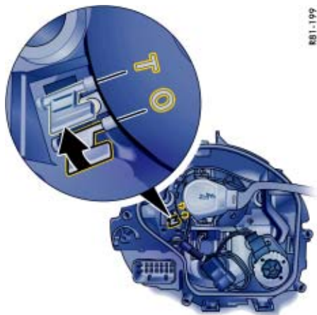
不带弯道灯的大灯
