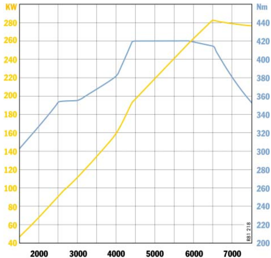
全负荷的发动机曲线图 - 911 Carrera S
