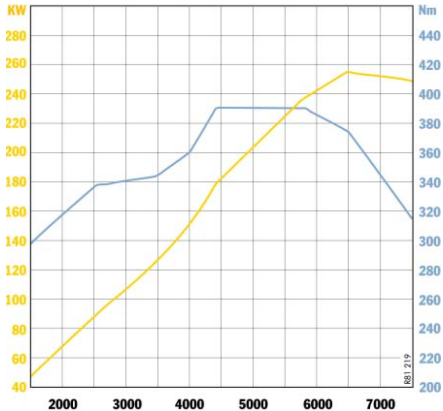
全负荷的发动机曲线图 - 911 Carrera
