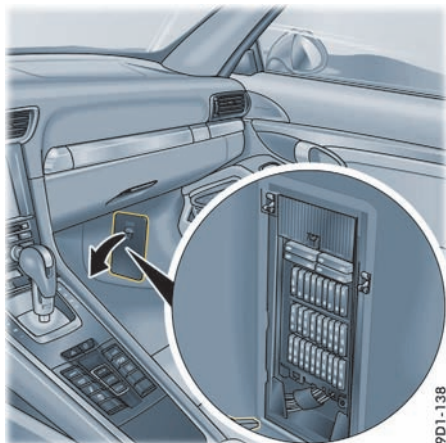
右侧脚坑中的保险丝
