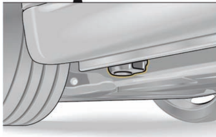
用于举升平台和千斤顶的前部举升点
