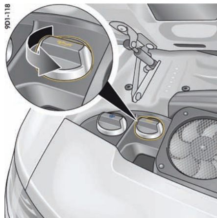
Coupé 机油加注点
