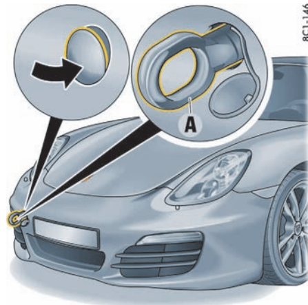
前牵引凸耳
