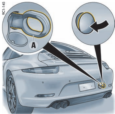
后牵引凸耳
