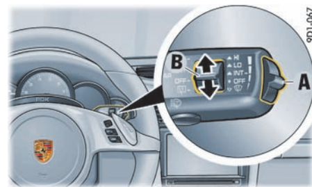
雨量传感器灵敏度开关 (A) 和后雨刷器开关 (B)
