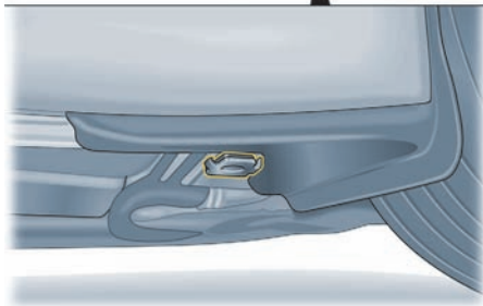
用于提升平台和千斤顶的后部举升点
