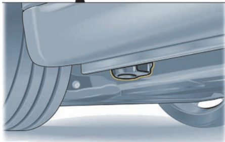
用于提升平台和千斤顶的前部举升点
