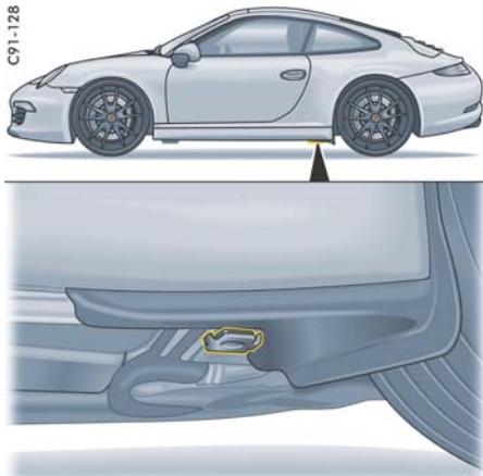
用于提升平台和千斤顶的后部举升点
